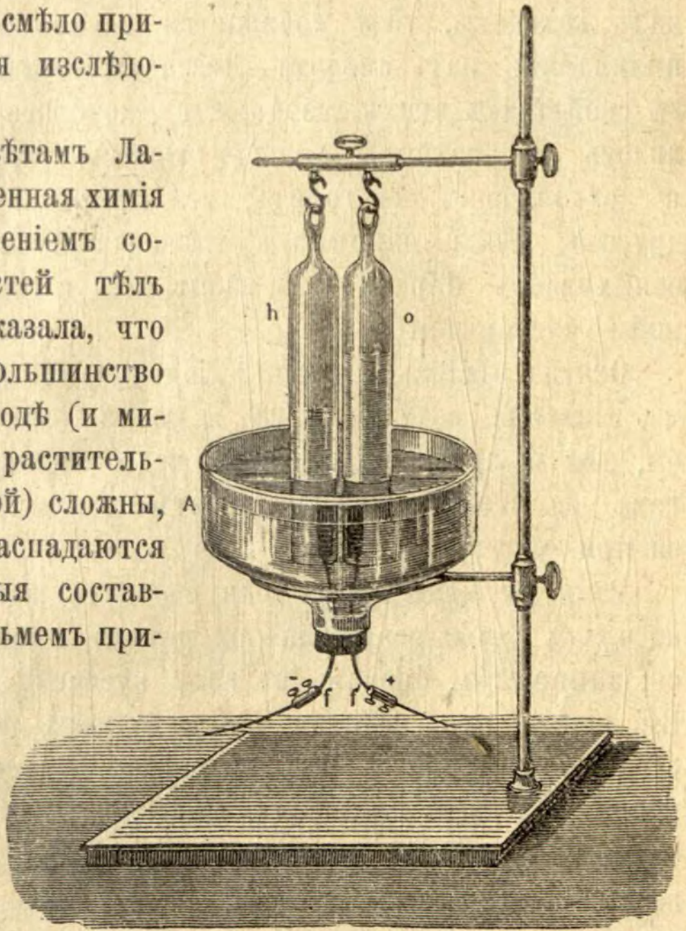
Рис. 3. Вольтаметръ. Приборъ для разложенія воды электрическимъ токомъ.
