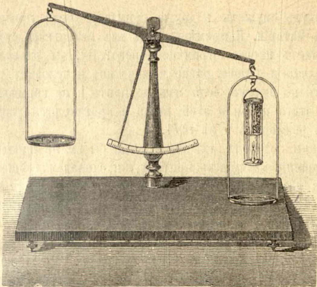
Рис. 1. Горѣніе свѣчи на вѣсахъ.
