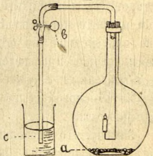
Рис. 2. Горѣніе свѣчи въ колбѣ, закрытой пробкой съ трубкой. а) Кусочки ѣдкаго натра; б) наружный зажимъ; в) подкрашенная вода.
