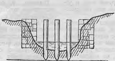
Если плотина длинная, придется вбить сваи, чтобы поддерживать доски.
